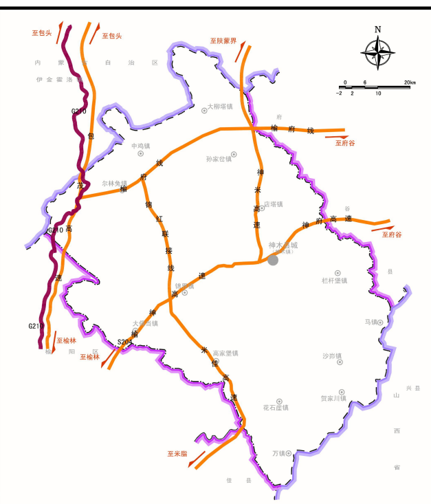
县域道路体系规划图
