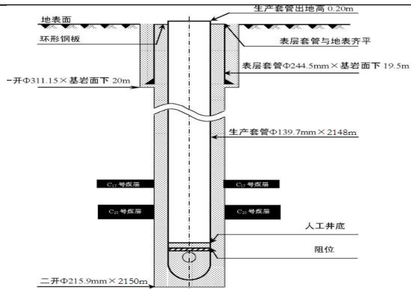
图 4 井身结构图
