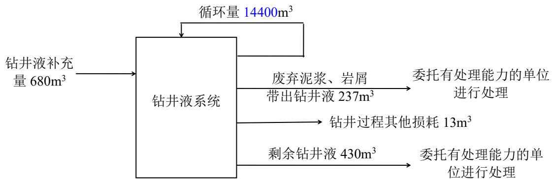
图2-1 钻井液循环量示意图
