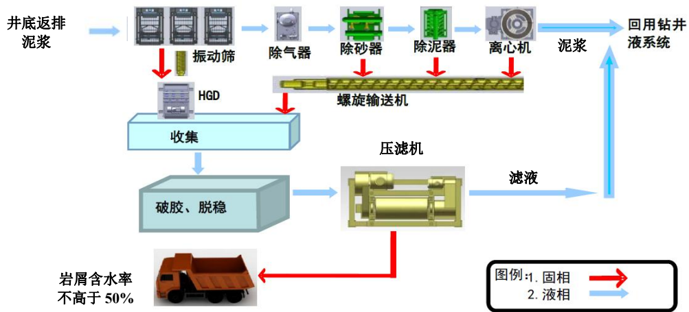
图 5 泥浆循环系统工艺流程简图
