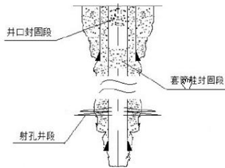
图 7 封井结构示意图
