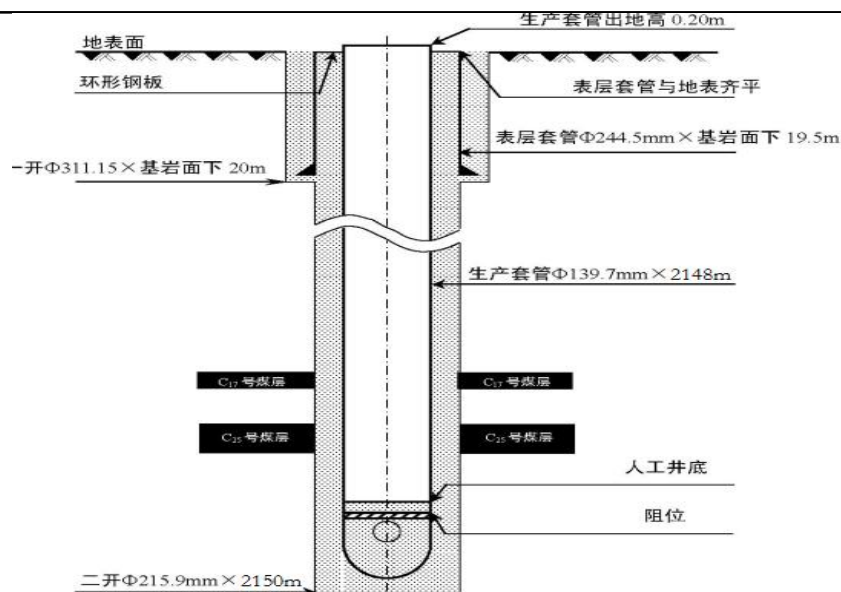
图 4 井身结构图
