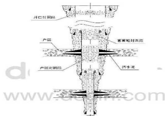
图 8 永久封井结构示意图
