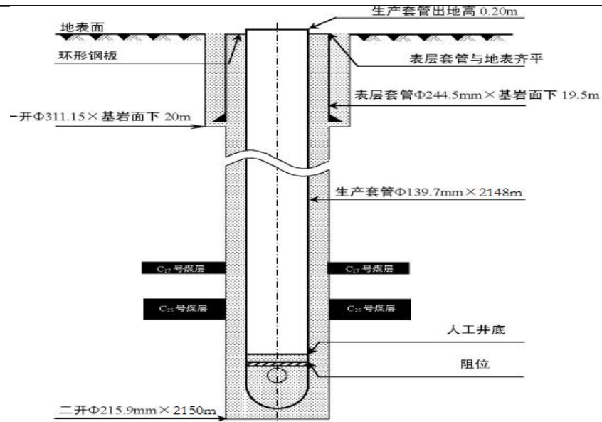
图 4 井身结构图
