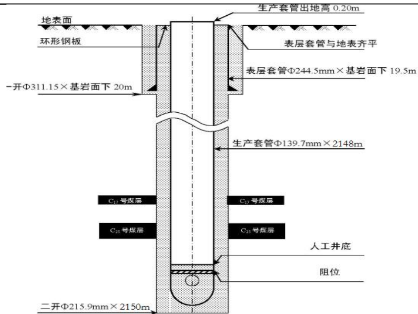
图 4 井身结构图
