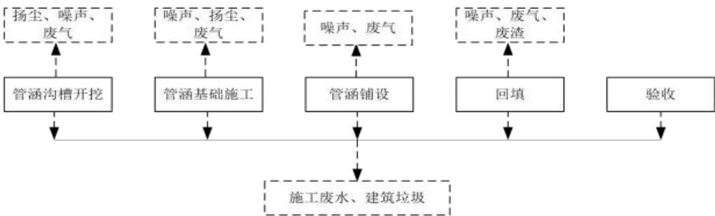
图 2-2 排水涵管工程施工期工艺流程及产污环节图
