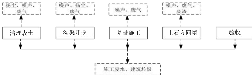
图 2-1 灌溉渠道工程施工期工艺流程及产污环节图
