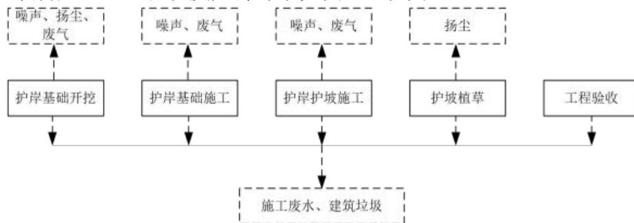
图 2-1 护岸工程施工期工艺流程及产污环节图
