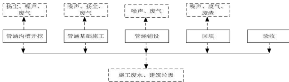
图 2-2 排水涵洞、涵管工程施工期工艺流程及产污环节图
