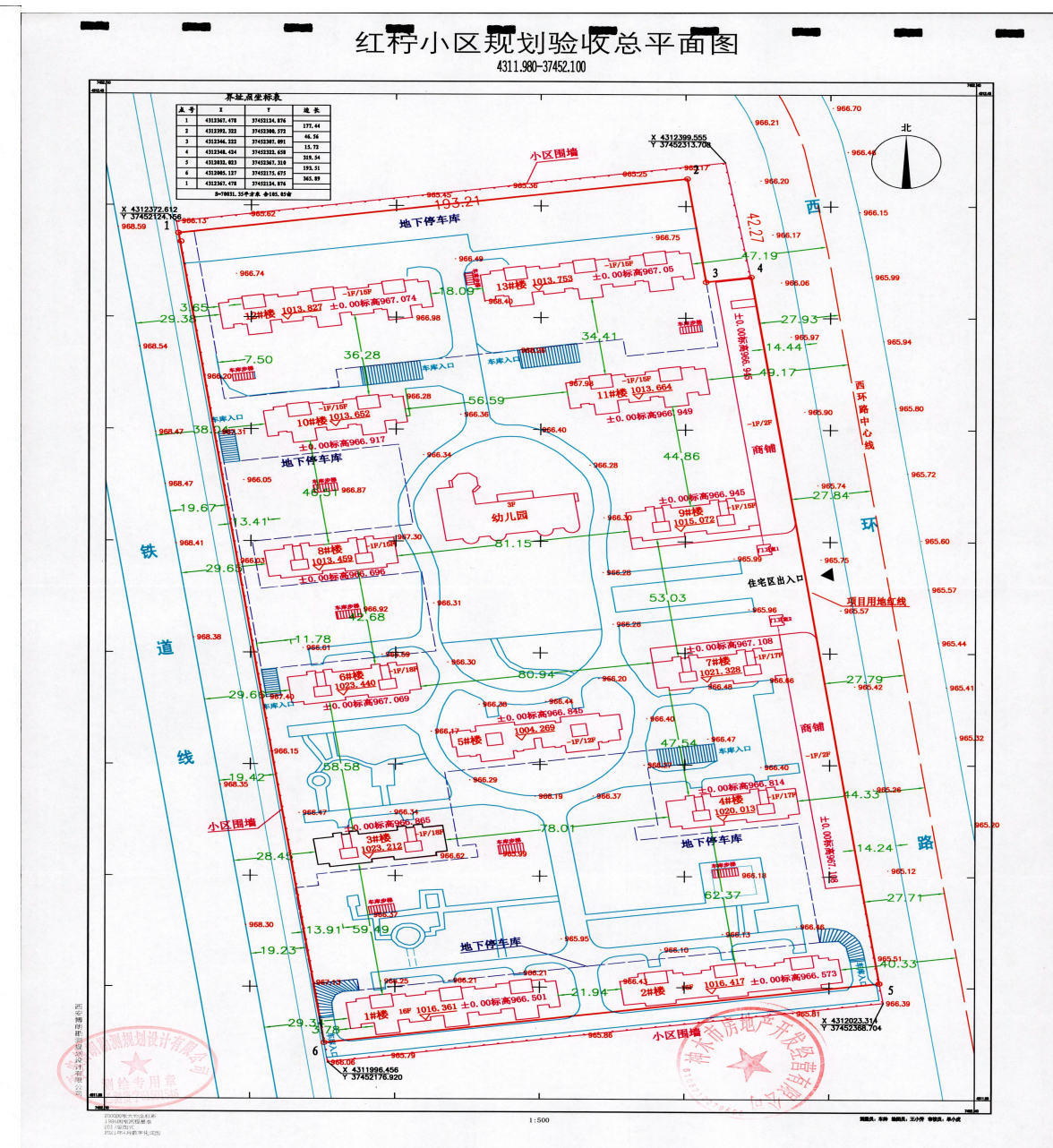
规划核实总平面图
