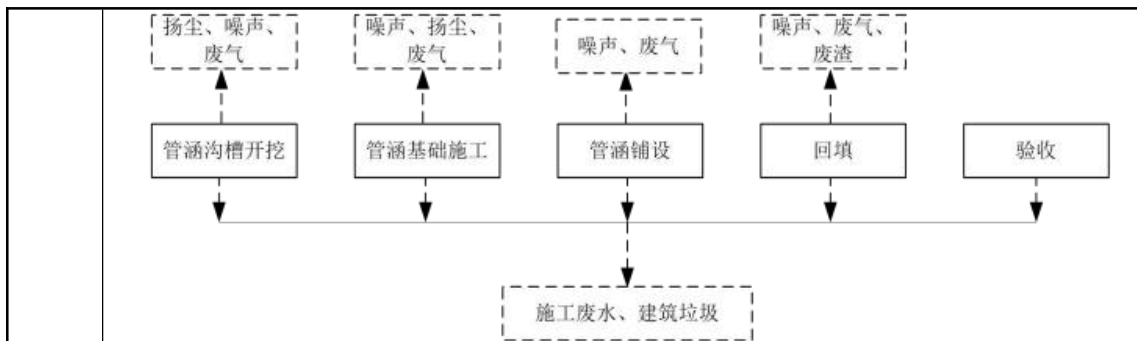
图 2-2 箱涵工程施工期工艺流程及产污环节图
