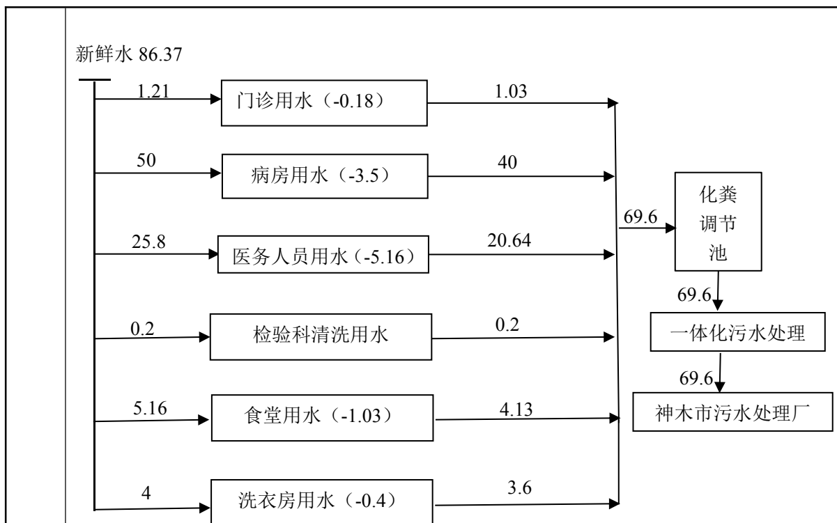
图 1 项目给排水平衡图 单位: m³/d
