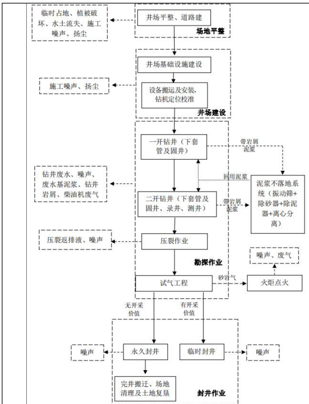
图 2-5 项目主要工艺流程及产污环节
