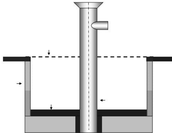
图 2-2 一开井口装置示意图
