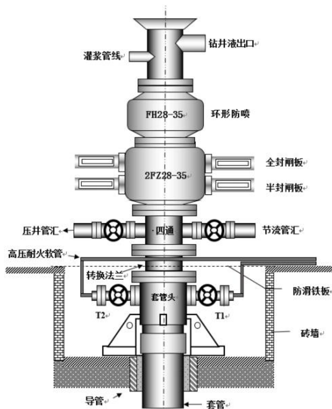
图 2-3 二开井口装置示意图
