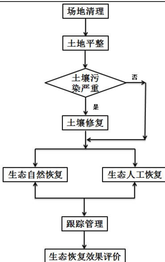
图 5-2 井场生态恢复步骤
