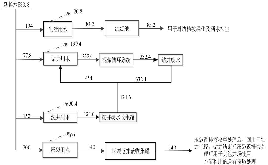
图 2-1 项目水平衡图 单位 m 3
