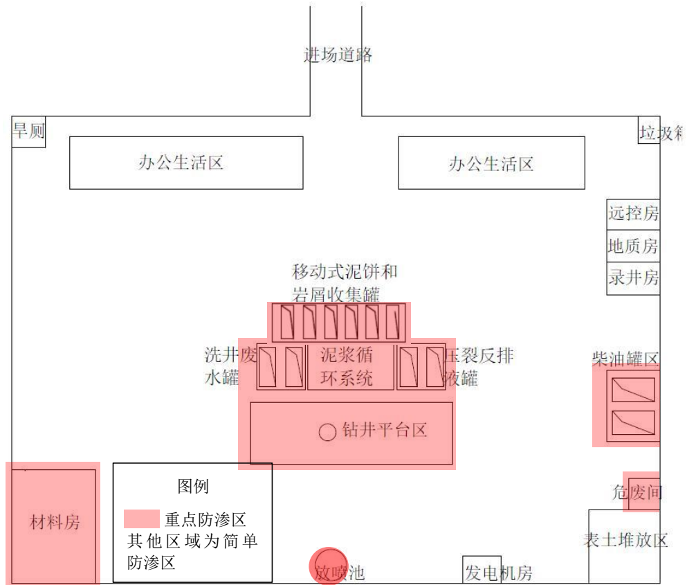
图 4-1 井场防渗分区图
